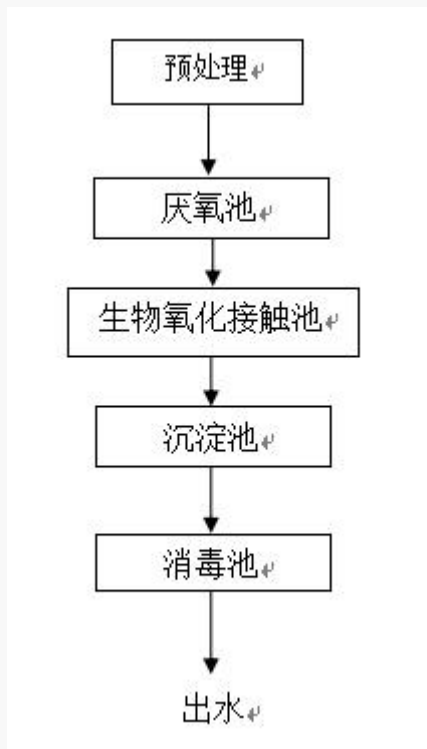
图3-3 污水处理工艺图
